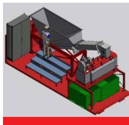
Paddle Depacker Model S de Mavitec como una solución en contenedores con un tamaño reducido.
