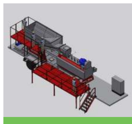
El Paddle Depacker Roadshow: una unidad de alquiler móvil para probar su propio material en su propio sitio.
