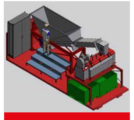
Küçük taban alanıyla, konteyner ile taşınan çözüm olarak Mavitec'in Paddle Depacker S Modeli.
