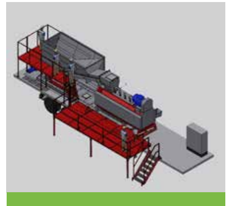
Paddle Depacker Mobil Ünite: Kendi malzemenizi kendi tesisinizde test etmek için kiralanabilir mobil ünite.
